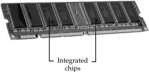
Fig. 1.13 RAM
