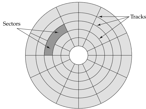
Fig. 1.15 Magnetic disk
