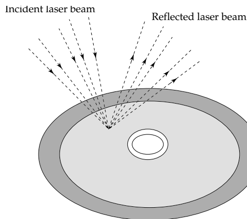
Fig. 1.16 Optical Disk
