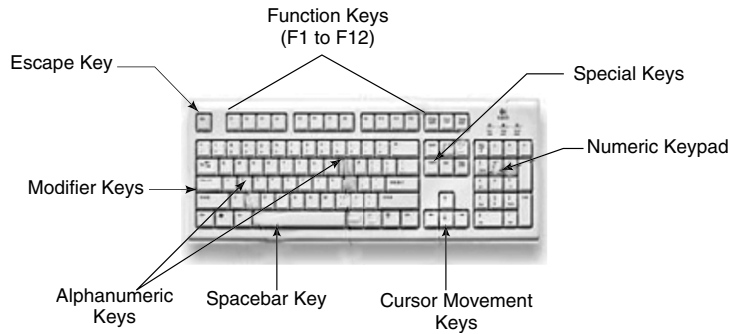
Fig. 1.4 Keyboard
